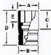
浅套筒
