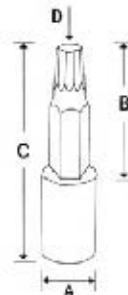
标准套筒螺丝刀头 短粗套筒螺丝刀头 加长套筒螺丝刀头
